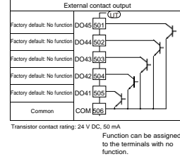
501-506 E4-Terminal Area
