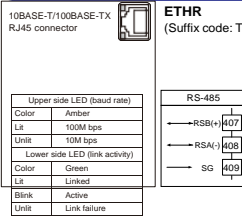
401-412 E3-Terminal Area
