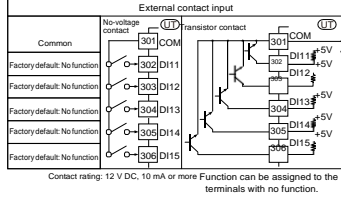
301-306 E1-Terminal Area
