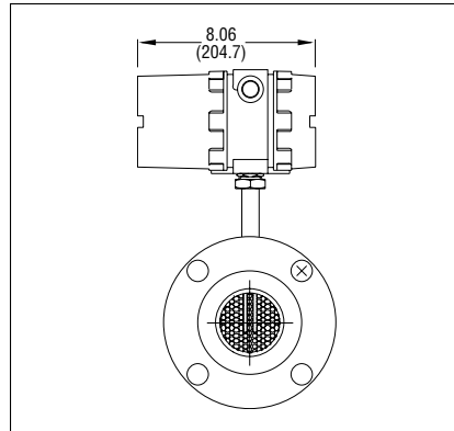
DIN Flange—Side View (E2)
