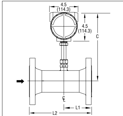
DIN Flange—Front View (E2)
