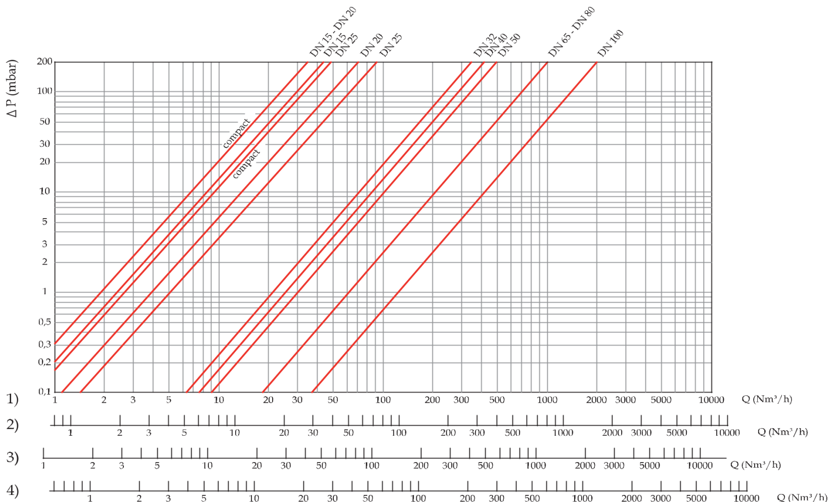
Diagramma perdite di carico - Capacity diagram - Diagramme pertes de charge - Diagrama de caudales
