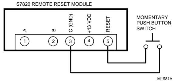
Fig. 3. Wiring Remote Reset Module.
